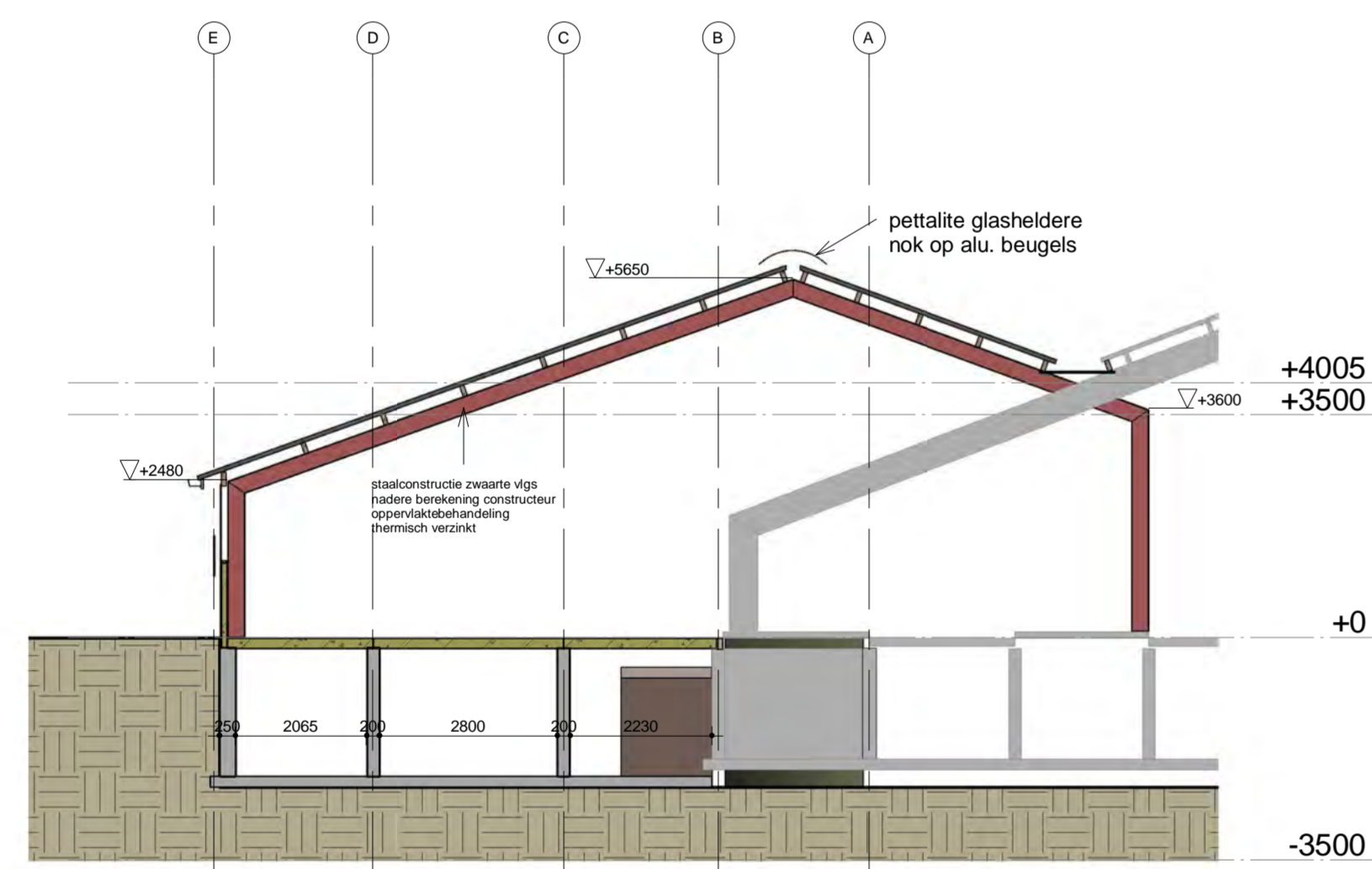
doorsnede A1
