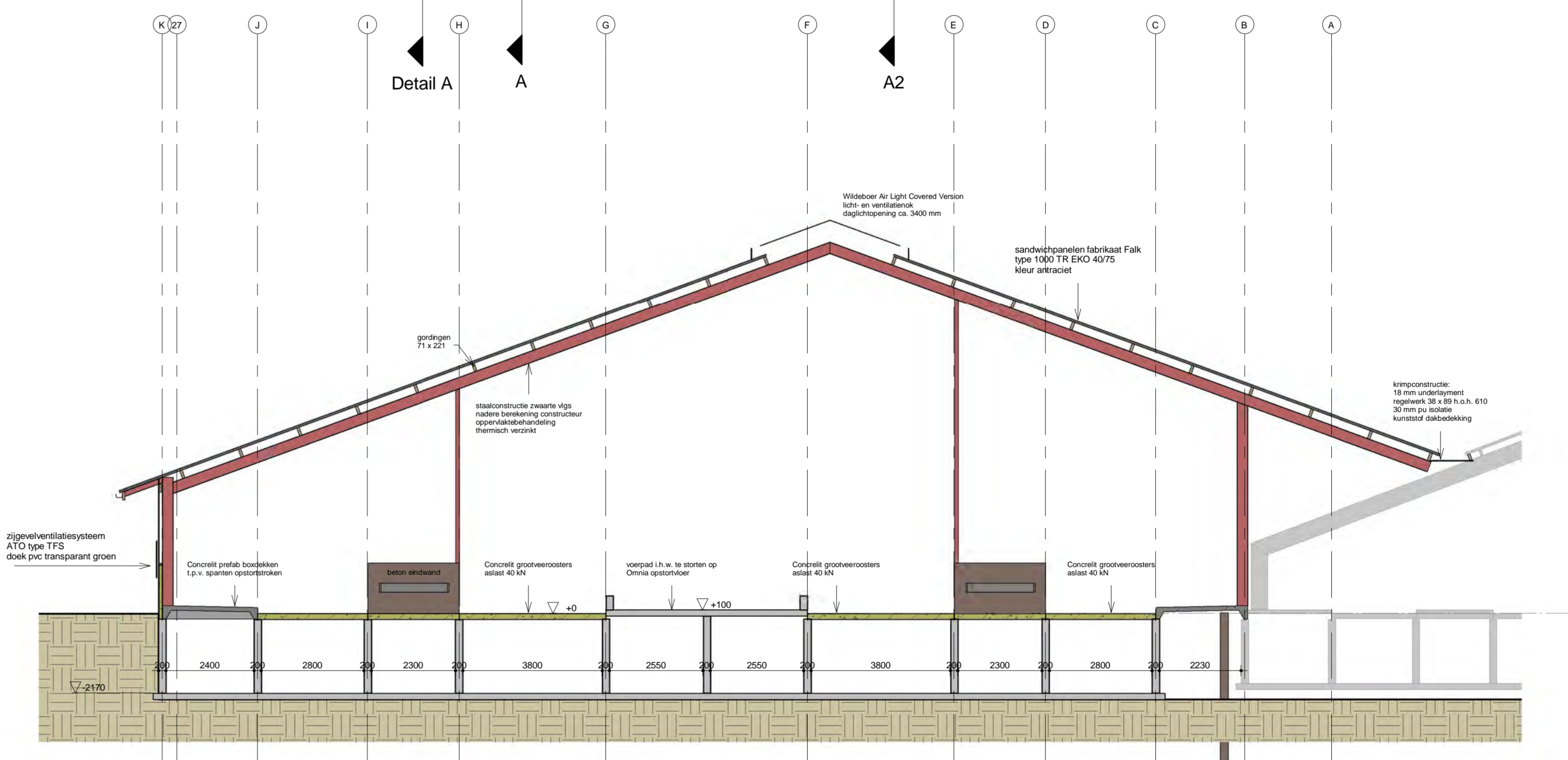
doorsnede A
